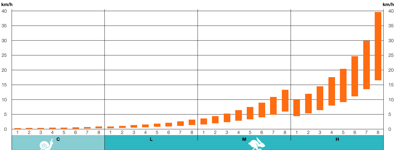
Velocità M6-121 U, M6-131 U, M6-141 U
